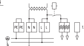
Schakelafbeelding Petr 30-U-Up-1
