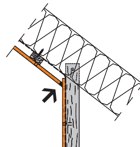
Afbeelding 15: Hoekaansluiting knieschot op kapbetimmering
